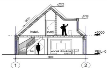
doorsnede A-A
